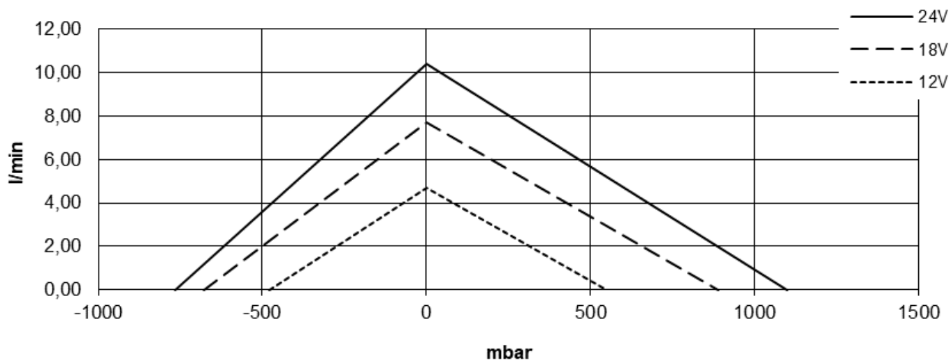
Type/Model: DC24/80KL
